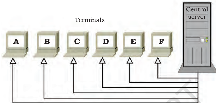
Fig. 4.23: Multi-user OS
