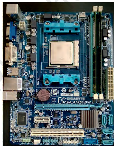
Fig. 7.6: FlexATX
